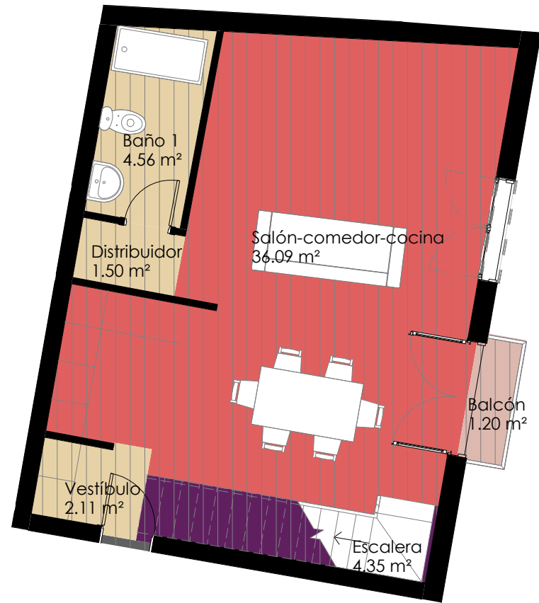
P1-1D-P.Primer 1:75
