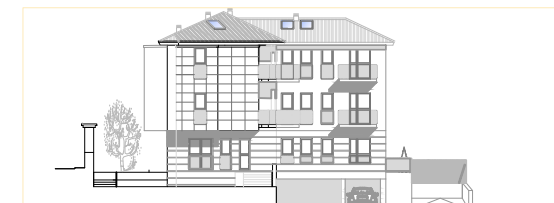
ALZADO SUR
